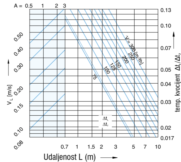
Brzina zraka uz zid - DK 200
