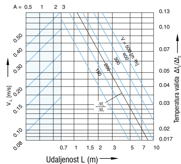
Brzina zraka uz zid - DK 315
