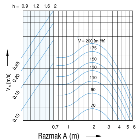
Raspored difuzora - DK 160 (u jednom ili više redova, ako je B ≥ 4,00 m)
