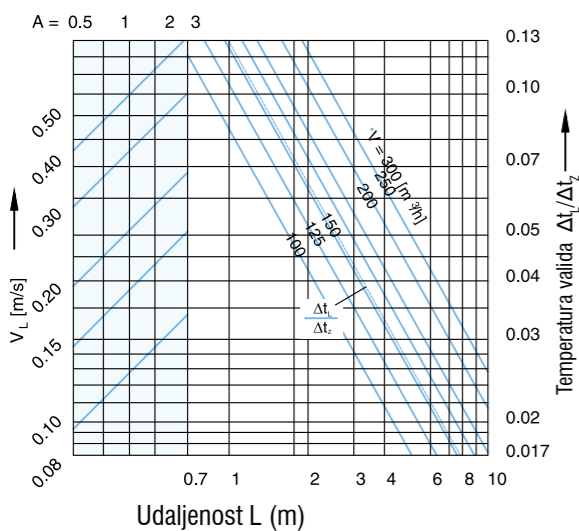
Brzina zraka uz zid - DK 250
