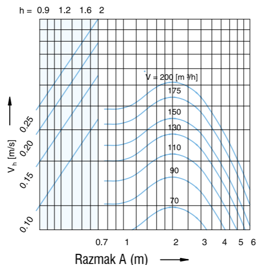
Raspored difuzora - DK 125 (u jednom ili više redova, ako je B ≥ 4,00 m)
