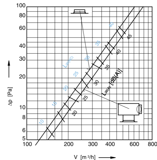
Dijagram razine buke i pada tlaka DK 315 - I
