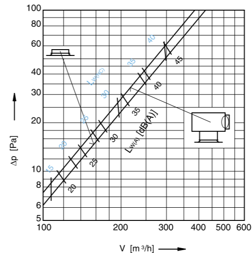
Dijagram razine buke i pada tlaka DK 200 - I
