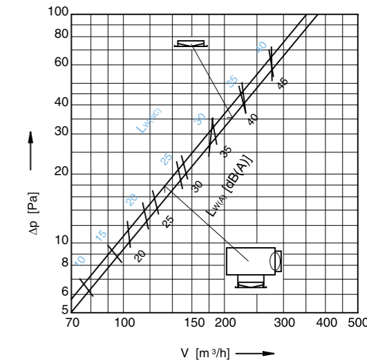
Dijagram razine buke i pada tlaka DK 250
