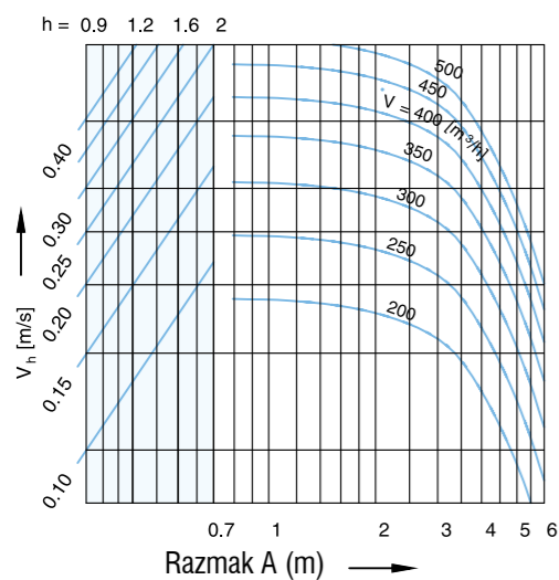
Raspored difuzora - DK 315 (u više od jednog reda, ako je B = 2,80 m)
