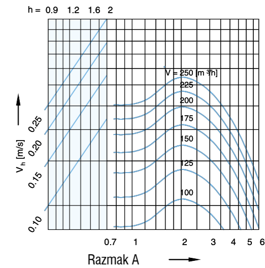
Kvadratni difuzor - DK 200
