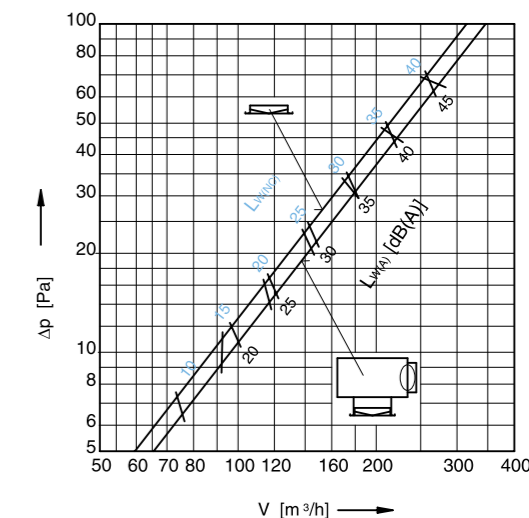
Dijagram razine buke i pada tlaka DK 200
