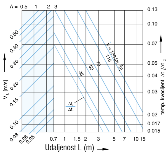
Brzina zraka uz zid - DK 125
