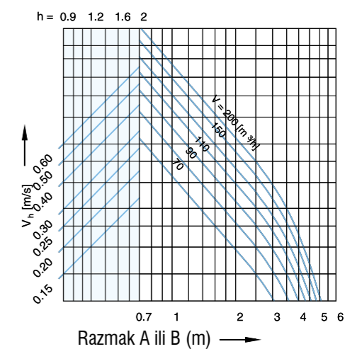
Brzina zraka uz zid - DK 160
