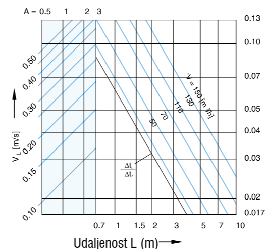
Brzina zraka uz zid - DK 160
