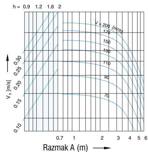
Raspored difuzora - DK 160 (u više od jednog reda, ako je B = 2,80 m)
