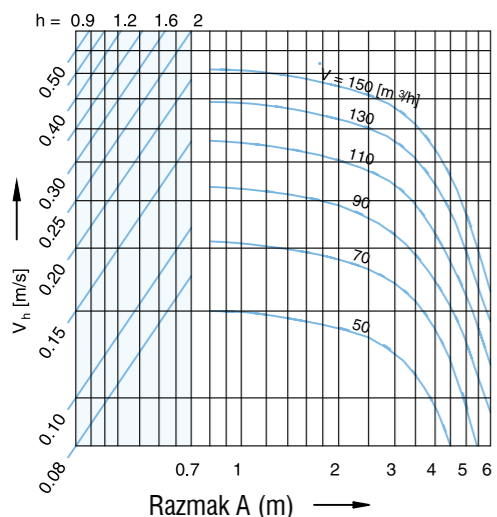
Raspored difuzora - DK 125 (u više od jednog reda, ako je B = 2,80 m)
