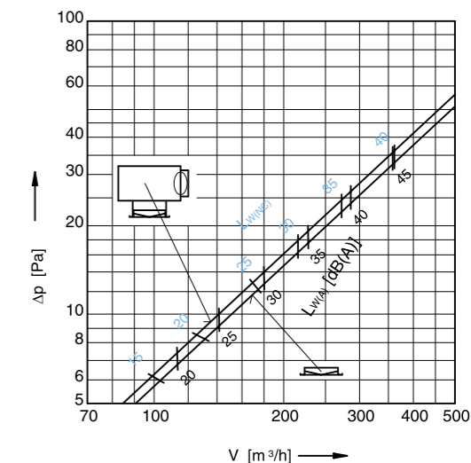
Dijagram razine buke i pada tlaka DK 315
