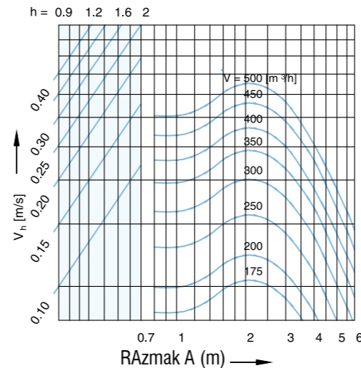
Raspored difuzora - DK 315 (u jednom ili više redova, ako je B ≥ 4,00 m)
