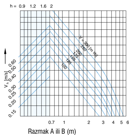
Kvadratni difuzor - DK 250
