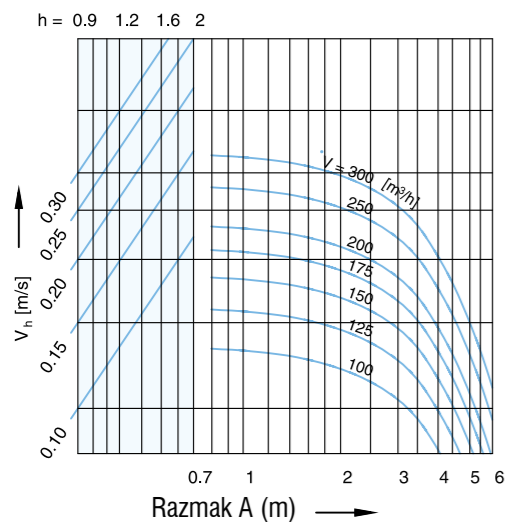
Brzina zraka uz zid - DK 250
